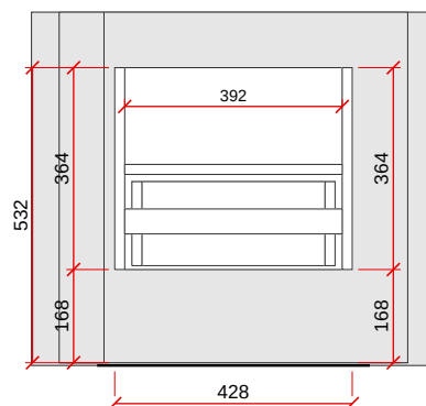
VISTA D - ESC. 1:15
